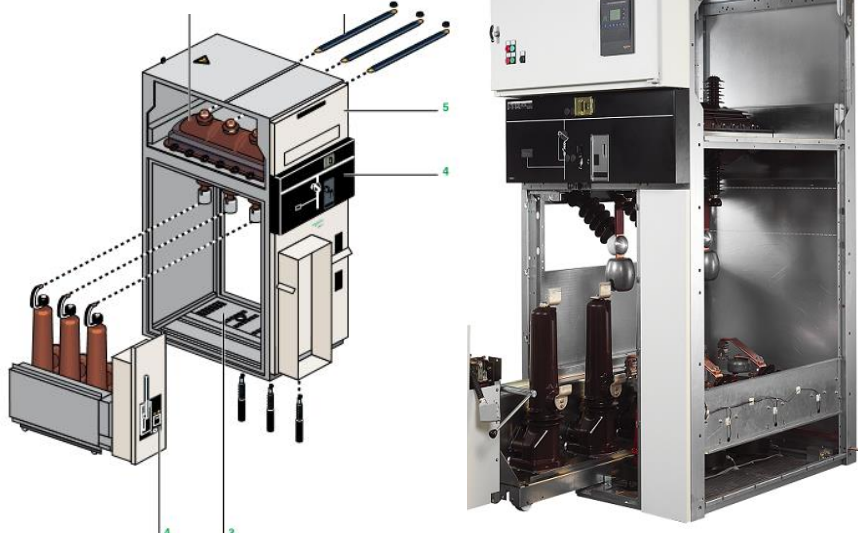
SM6 Sabit/Çekmeceli OG Hücreler
